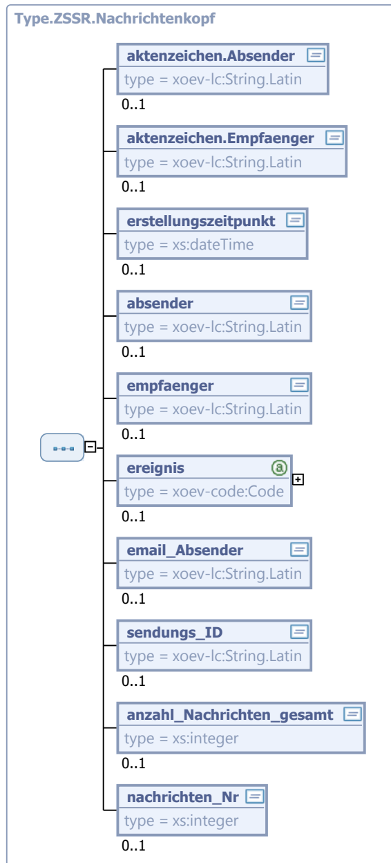
Abbildung 22.4. Type.ZSSR.Nachrichtenkopf
