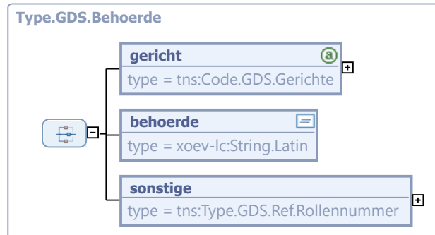
Abbildung 4.14. Type.GDS.Behoerde
