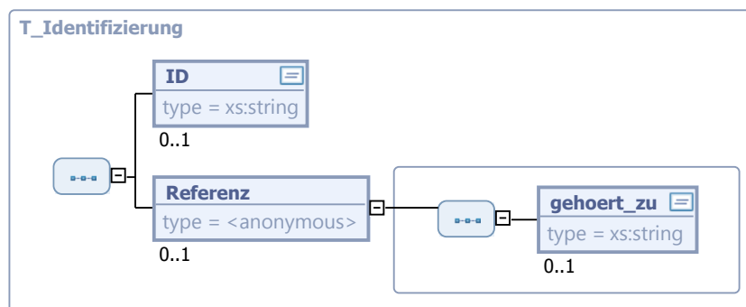
Abbildung 4.63. T_Identifizierung
