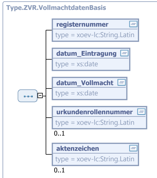
Abbildung 13.5. Type.ZVR.VollmachtdatenBasis
