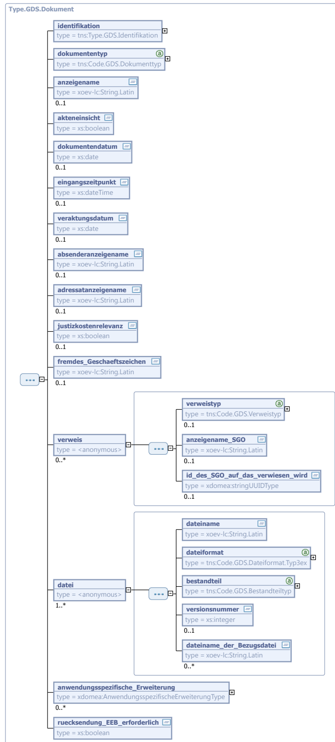
Abbildung 4.18. Type.GDS.Dokument
