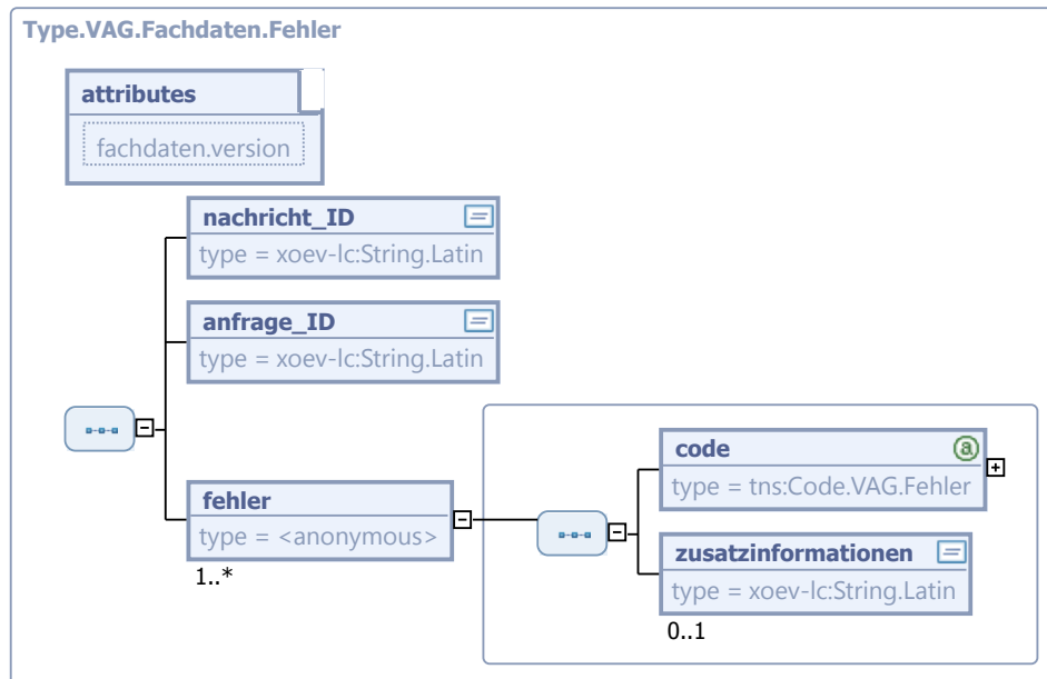
Abbildung 6.6. Type.VAG.Fachdaten.Fehler
