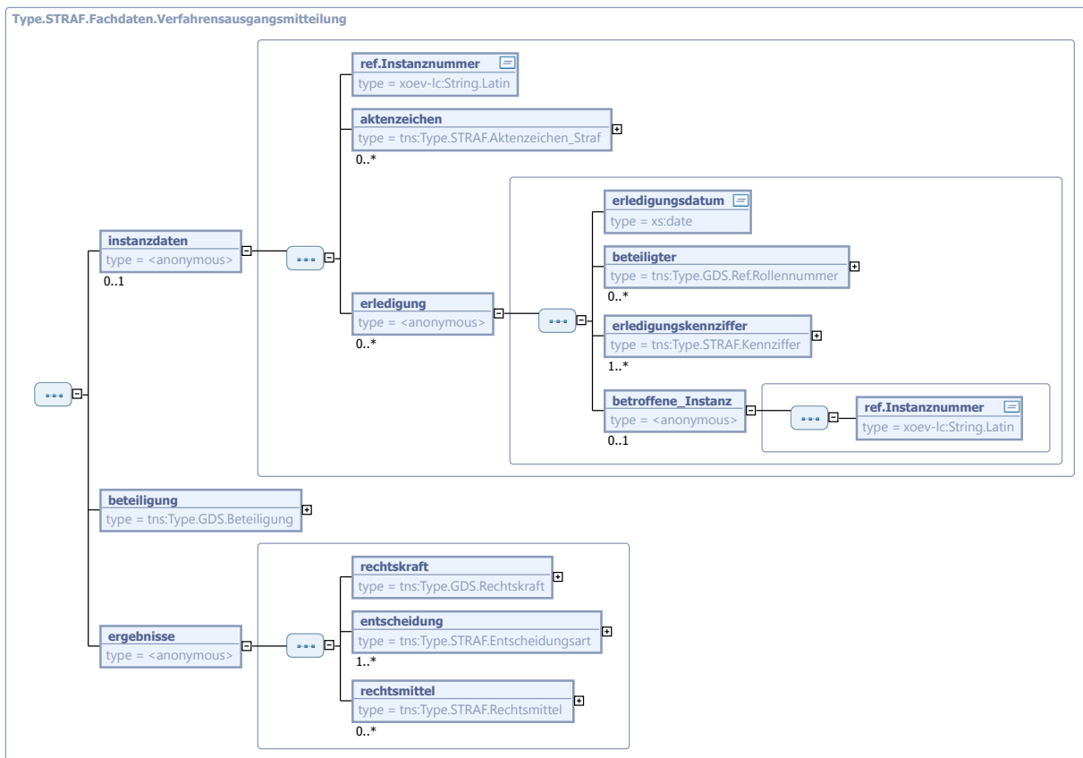
Abbildung 9.11. Type.STRAF.Fachdaten.Verfahrensausgangsmittelung
