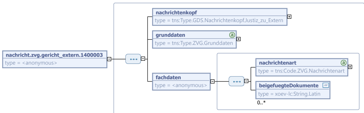
Abbildung 15.4. nachricht.zvg.gericht_extern.1400003
