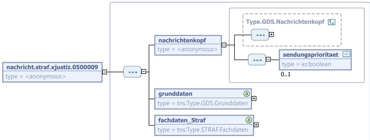
Abbildung 9.31. nachricht.straf.xjustiz.0500009
