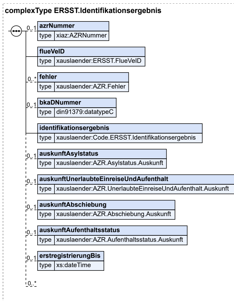
Abbildung 13.52. ERSST.Identifikationsergebnis
