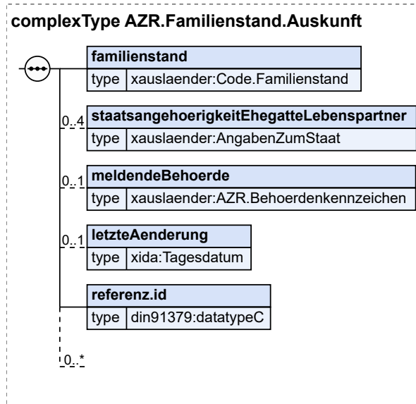
Abbildung 8.77. AZR.Familienstand.Auskunft
