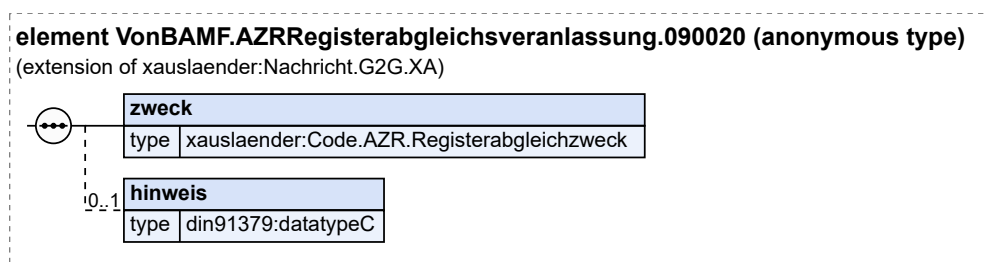
Abbildung 8.27. VonBAMF.AZRRegisterabgleichsveranlassung.090020
