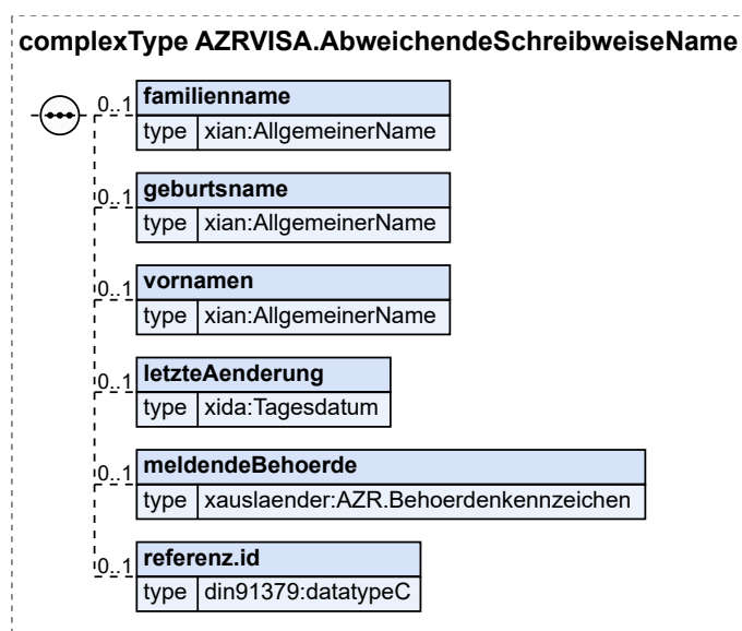
Abbildung 8.219. AZRVISA.AbweichendeSchreibweiseName
