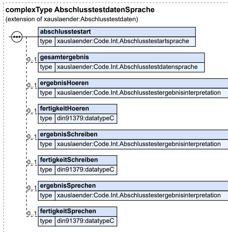
Abbildung 7.6. AbschlusstestdatenSprache
