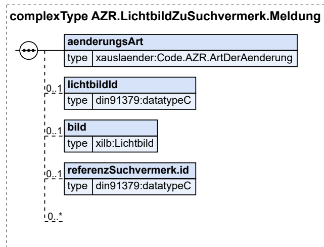
Abbildung 8.161. AZR.LichtbildZuSuchvermerk.Meldung
