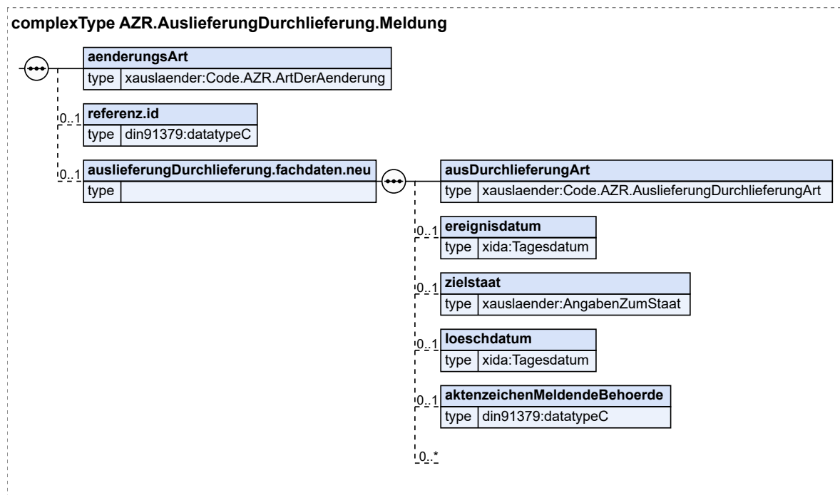
Abbildung 8.132. AZR.AuslieferungDurchlieferung.Meldung
