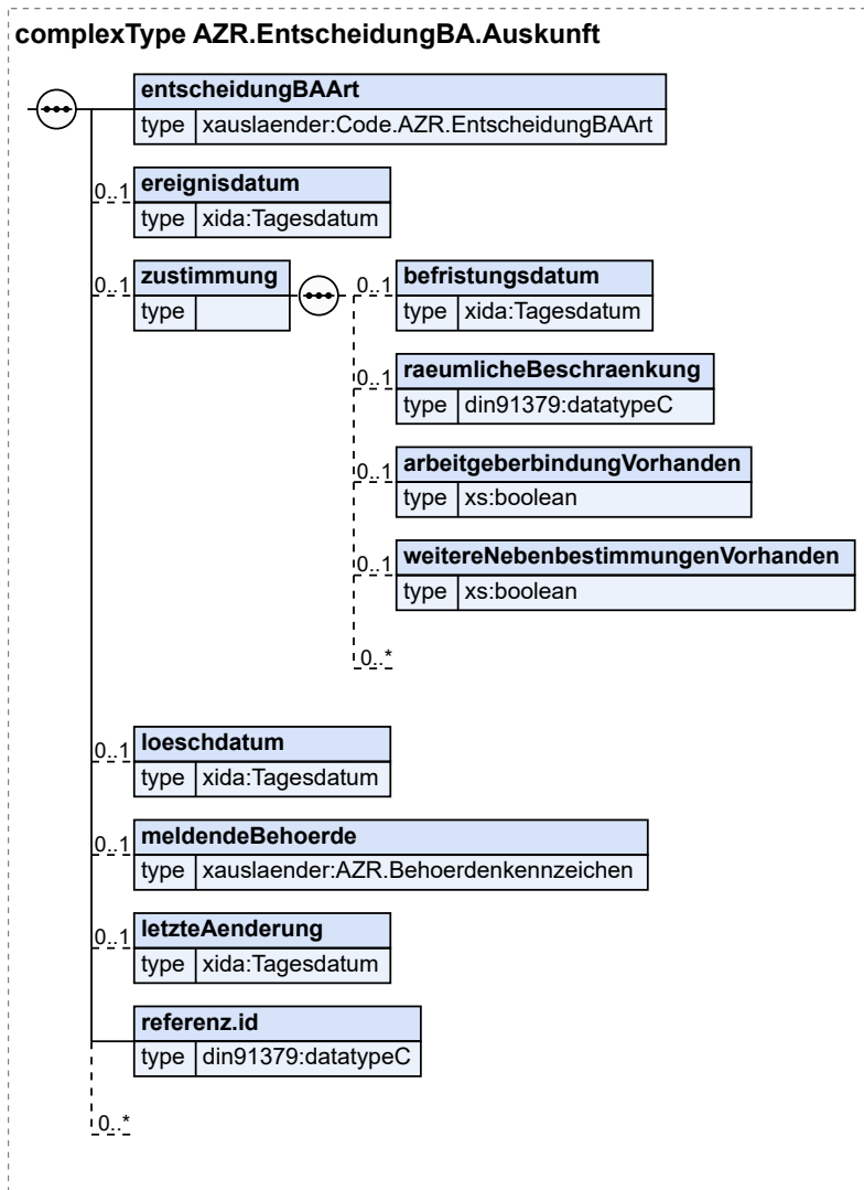
Abbildung 8.74. AZR.EntscheidungBA.Auskunft
