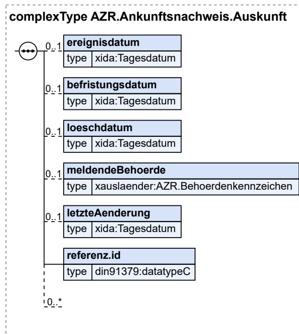
Abbildung 8.50. AZR.Ankunftsnachweis.Auskunft
