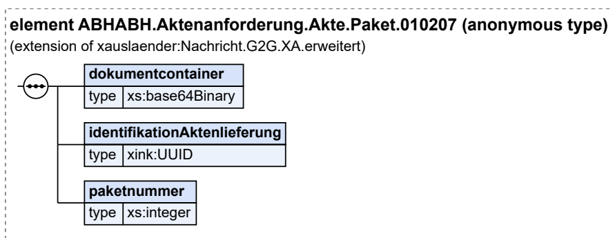
Abbildung 3.14. ABHABH.Aktenanforderung.Akte.Paket.010207
