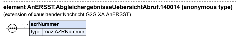
Abbildung 13.31. AnERSST.AbgleichergebnisseUebersichtAbruf.140014
