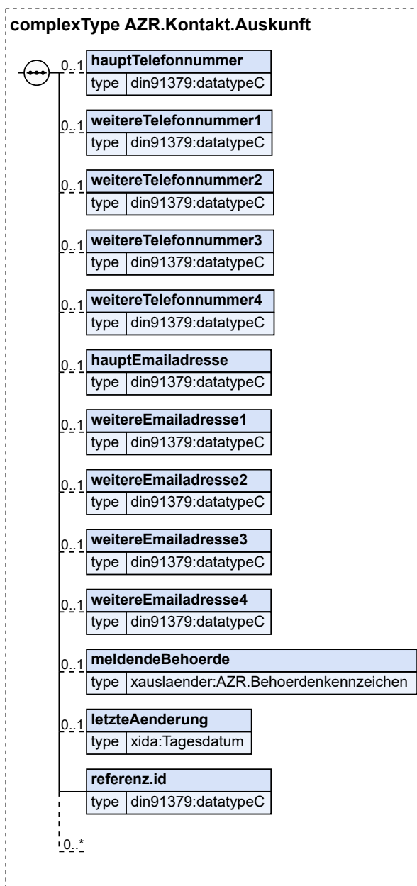
Abbildung 8.85. AZR.Kontakt.Auskunft
