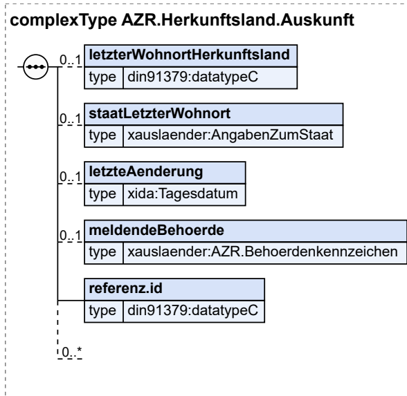
Abbildung 8.83. AZR.Herkunftsland.Auskunft
