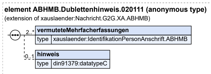
Abbildung 4.15. ABHMB.Dublettenhinweis.020111
