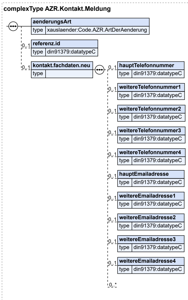
Abbildung 8.159. AZR.Kontakt.Meldung
