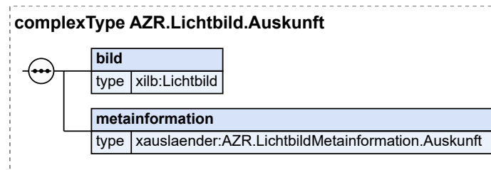
Abbildung 8.86. AZR.Lichtbild.Auskunft
