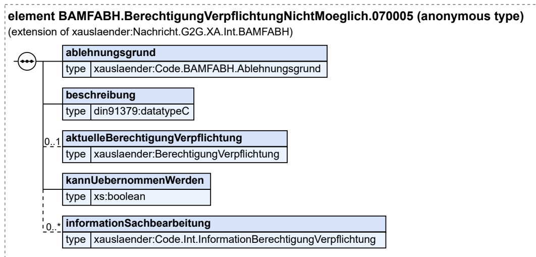
Abbildung 6.26. BAMFABH.BerechtigungVerpflichtungNichtMoeglich.070005
