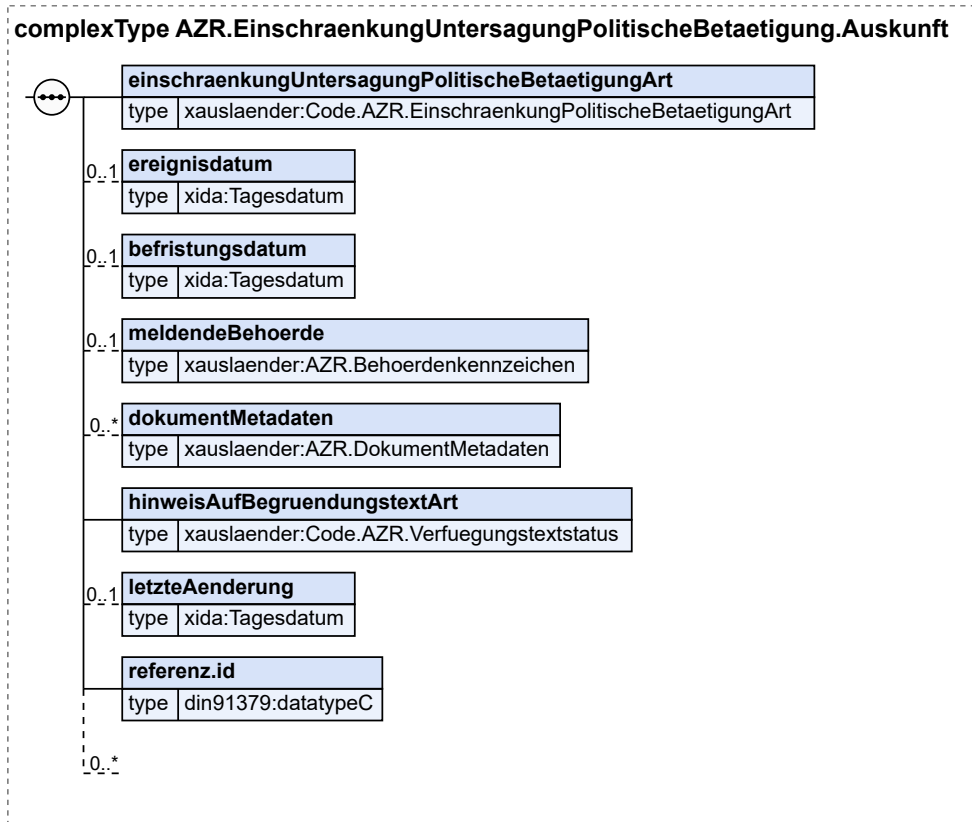
Abbildung 8.73. AZR.EinschraenkungUntersagungPolitischeBetaetigung.Auskunft
