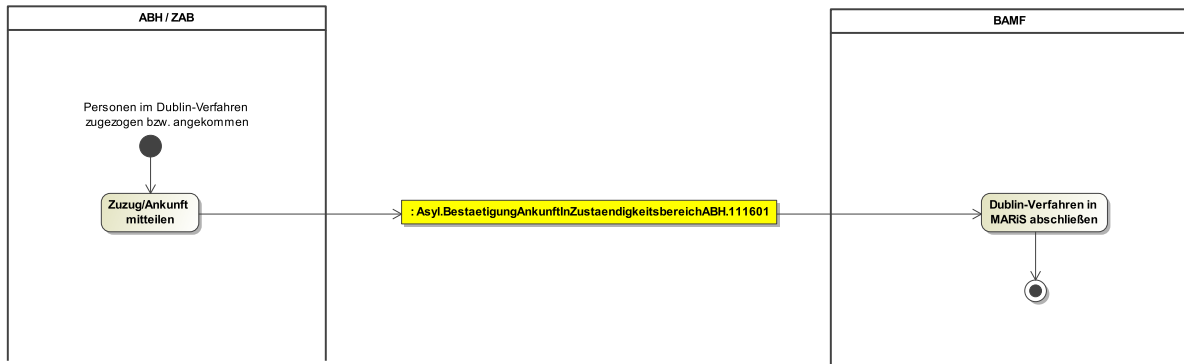
Abbildung 10.40. Dublin-Verfahren Zuzug/Ankunft
