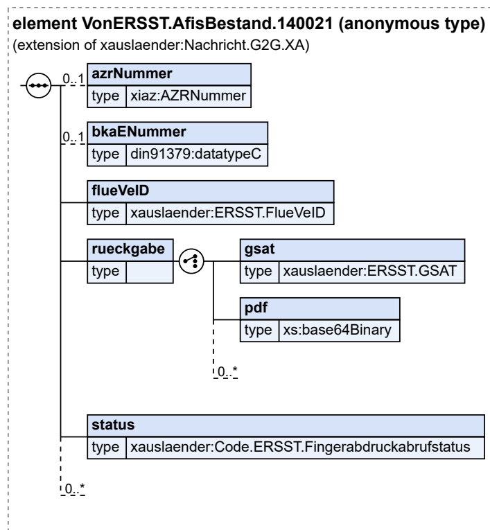
Abbildung 13.38. VonERSST.AfisBestand.140021
