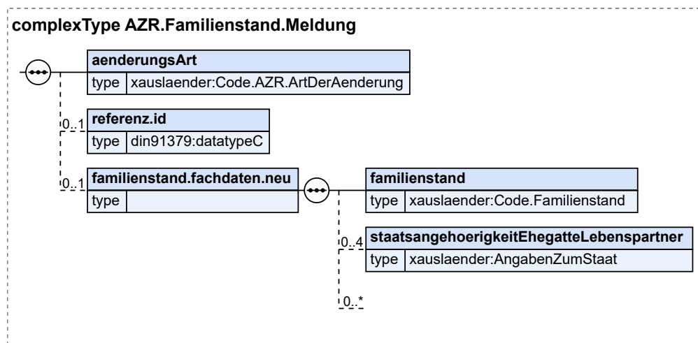
Abbildung 8.150. AZR.Familienstand.Meldung
