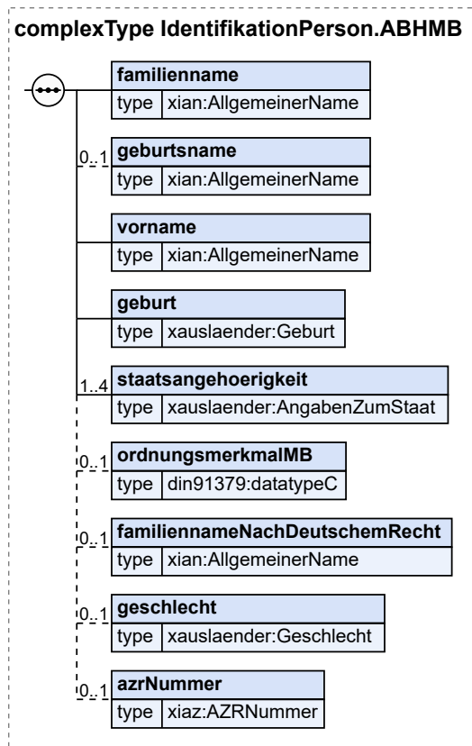
Abbildung 4.5. IdentifikationPerson.ABHMB
