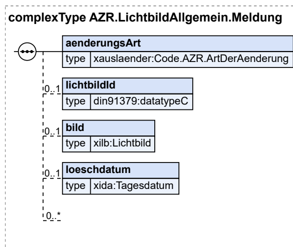
Abbildung 8.160. AZR.LichtbildAllgemein.Meldung
