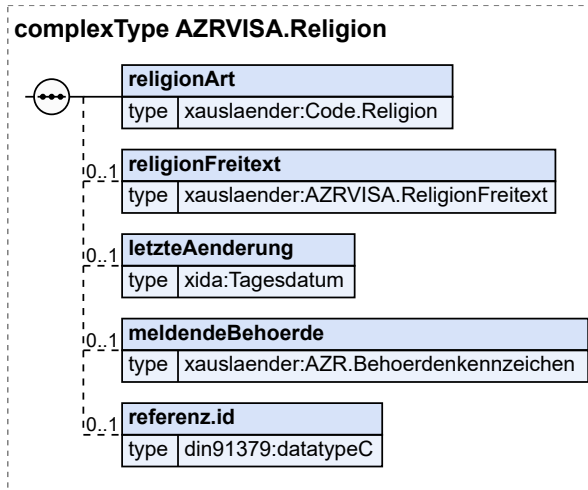
Abbildung 8.230. AZRVISA.Religion
