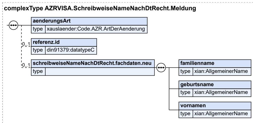
Abbildung 8.248. AZRVISA.SchreibweiseNameNachDtRecht.Meldung
