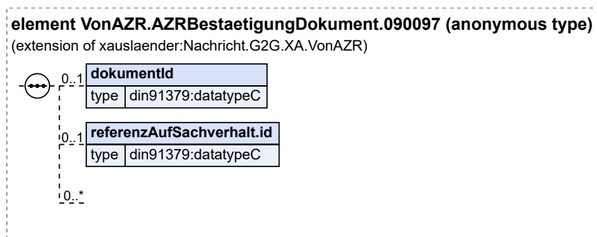
Abbildung 8.26. VonAZR.AZRBestaetigungDokument.090097
