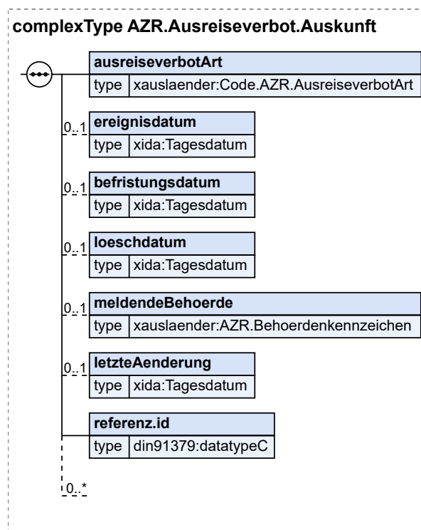
Abbildung 8.62. AZR.Ausreiseverbot.Auskunft
