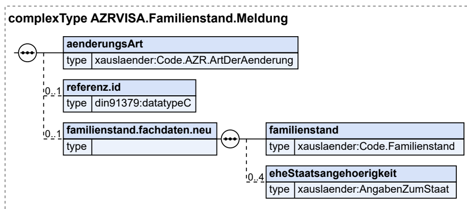
Abbildung 8.241. AZRVISA.Familienstand.Meldung
