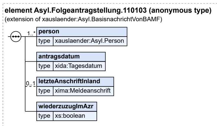
Abbildung 10.49. Asyl.Folgeantragstellung.110103
