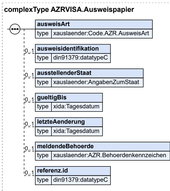
Abbildung 8.214. AZRVISA.Ausweispapier
