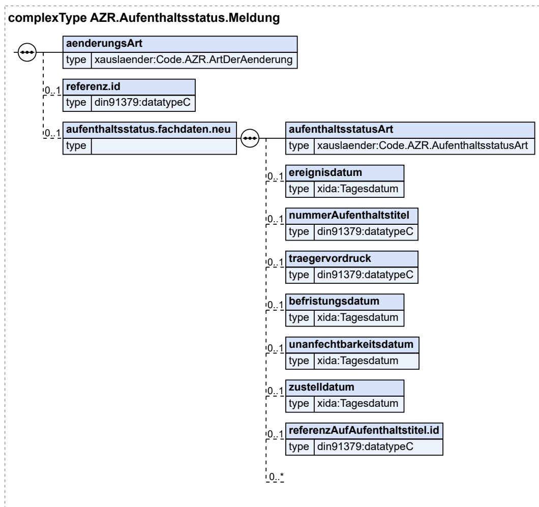
Abbildung 8.130. AZR.Aufenthaltsstatus.Meldung
