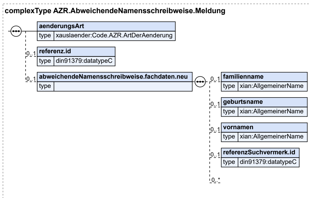
Abbildung 8.119. AZR.AbweichendeNamensschreibweise.Meldung
