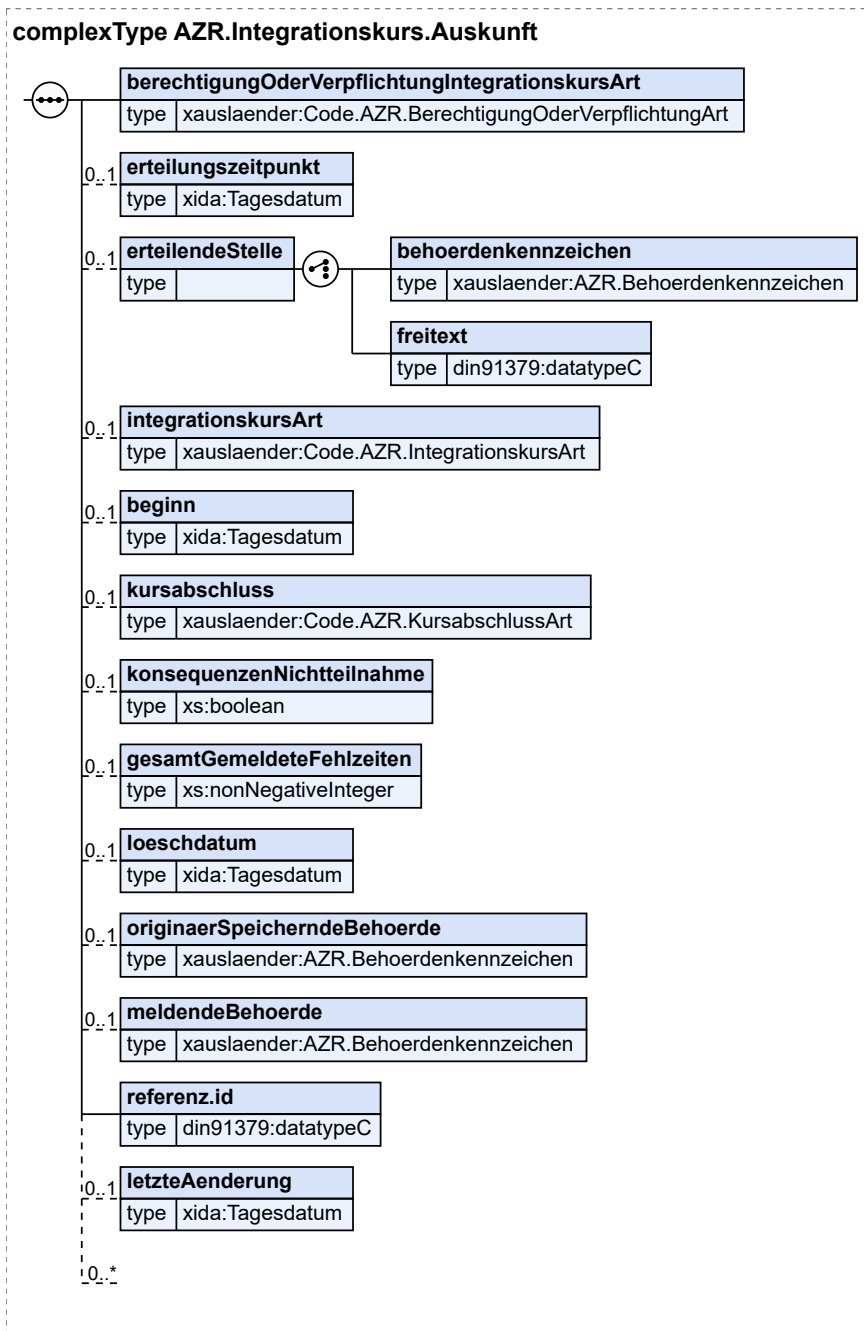
Abbildung 8.84. AZR.Integrationskurs.Auskunft
