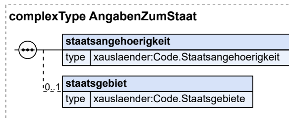
Abbildung 2.16. AngabenZumStaat
