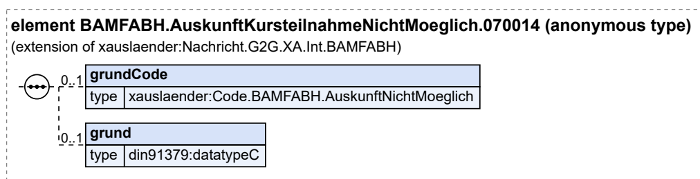
Abbildung 6.42. BAMFABH.AuskunftKursteilnahmeNichtMoeglich.070014
