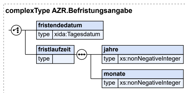
Abbildung 8.38. AZR.Befristungsangabe
