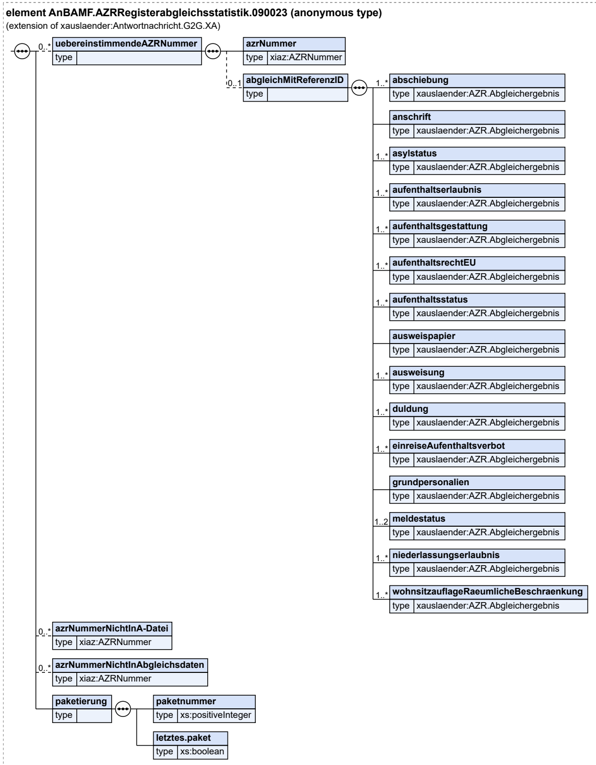
Abbildung 8.30. AnBAMF.AZRRegisterabgleichsstatistik.090023
