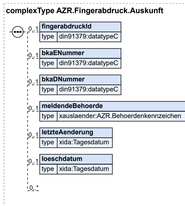
Abbildung 8.76. AZR.Fingerabdruck.Auskunft
