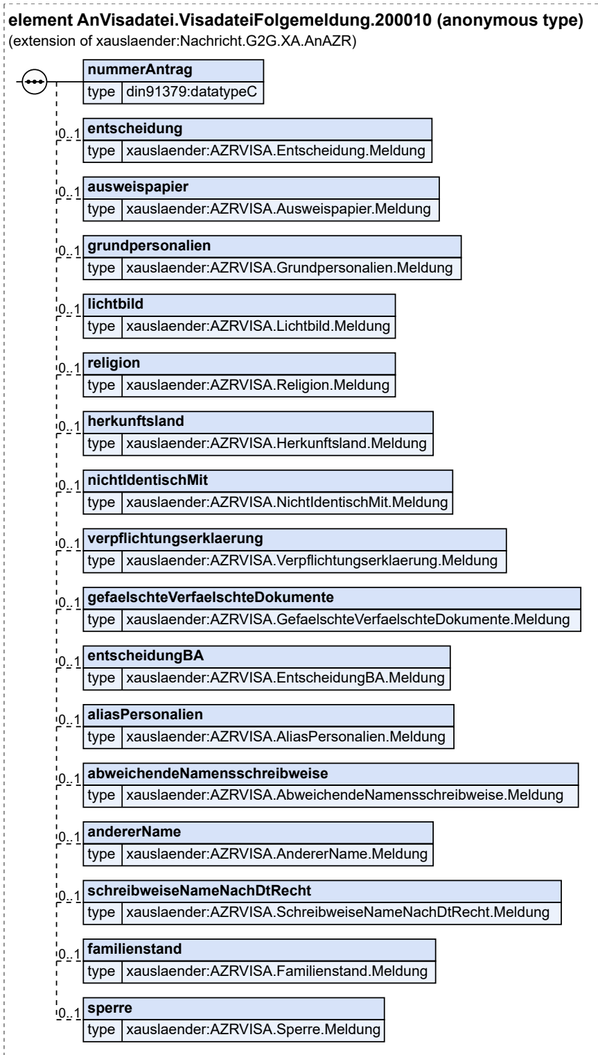
Abbildung 8.203. AnVisadatei.VisadateiFolgemeldung.200010
