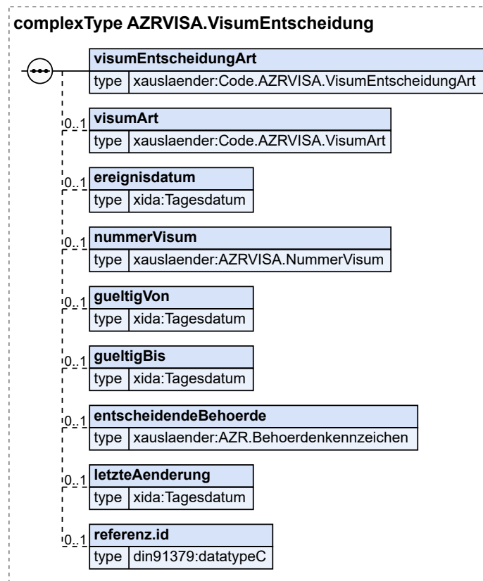
Abbildung 8.233. AZRVISA.VisumEntscheidung
