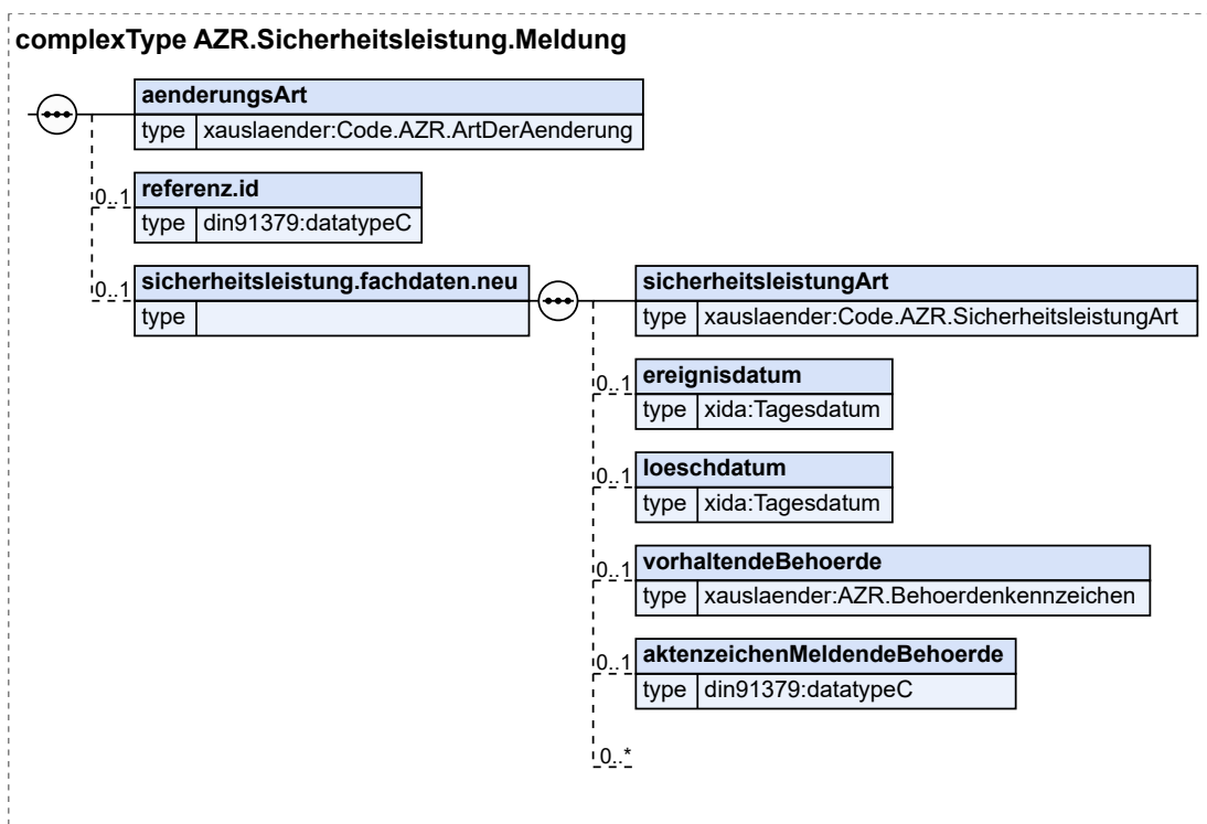
Abbildung 8.170. AZR.Sicherheitsleistung.Meldung
