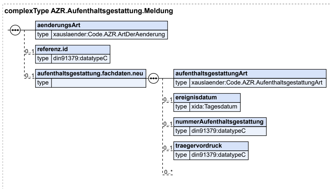
Abbildung 8.128. AZR.Aufenthaltsgestattung.Meldung
