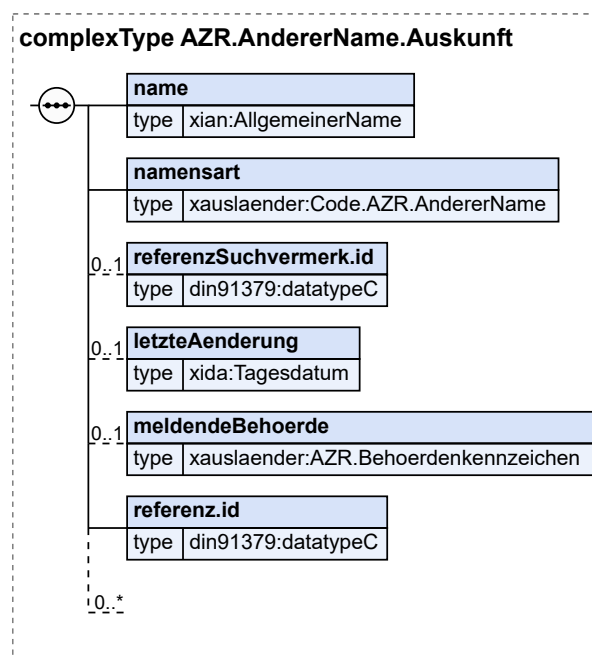
Abbildung 8.48. AZR.AndererName.Auskunft
