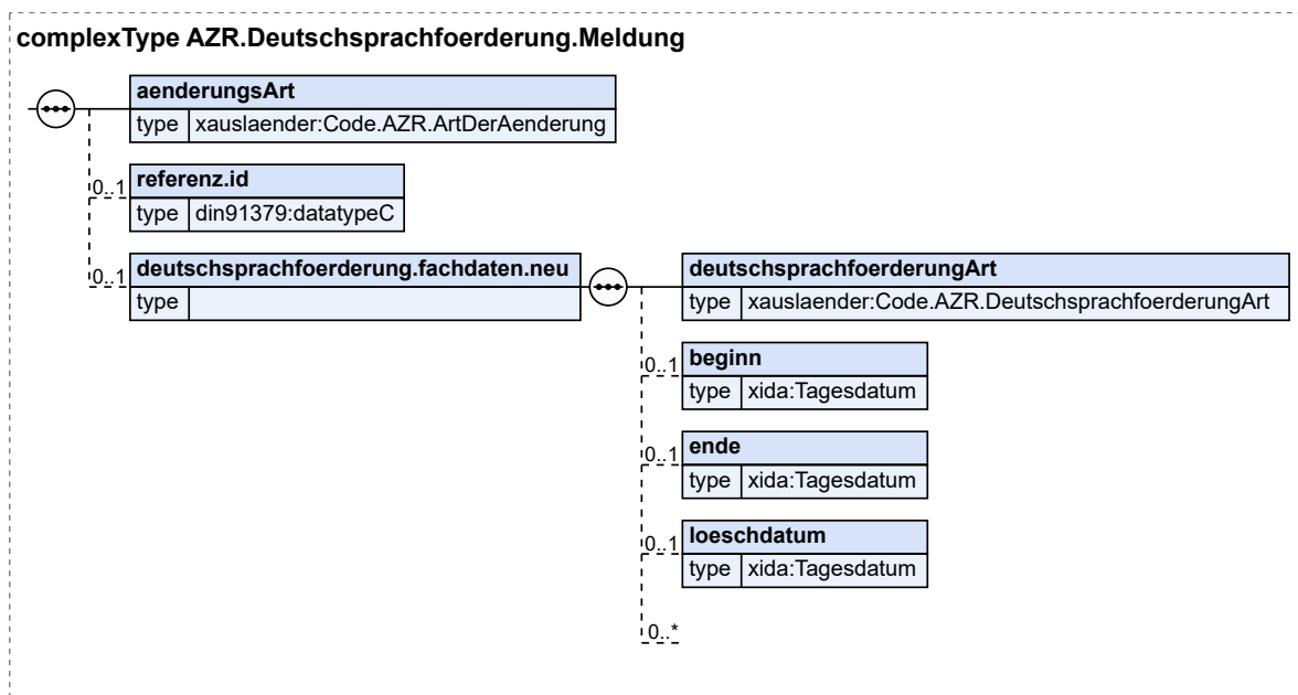
Abbildung 8.143. AZR.Deutschsprachfoerderung.Meldung
