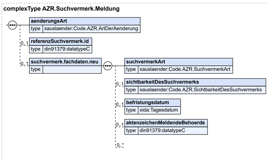
Abbildung 8.173. AZR.Suchvermerk.Meldung
