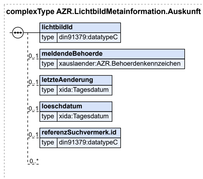
Abbildung 8.87. AZR.LichtbildMetainformation.Auskunft
