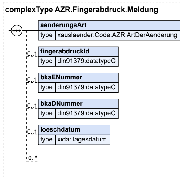
Abbildung 8.152. AZR.Fingerabdruck.Meldung
