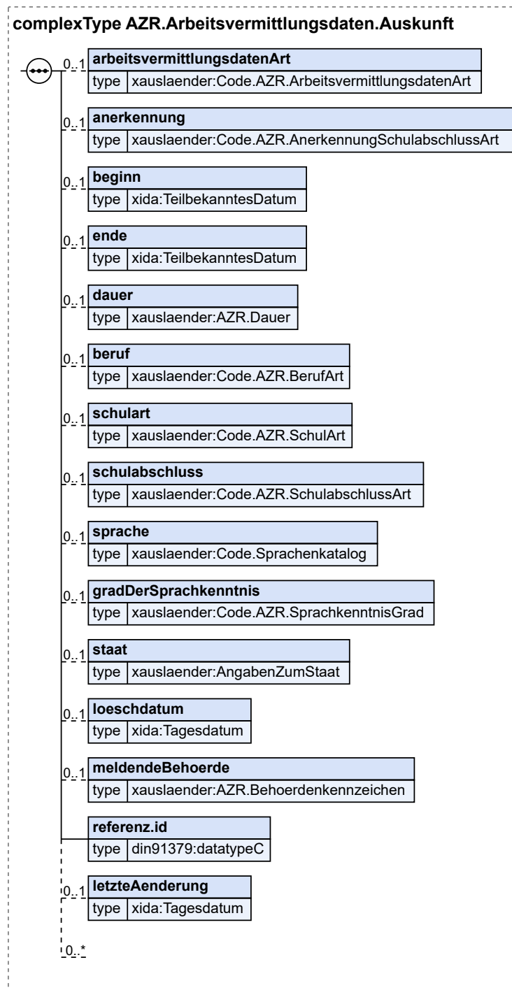
Abbildung 8.52. AZR.Arbeitsvermittlungsdaten.Auskunft
