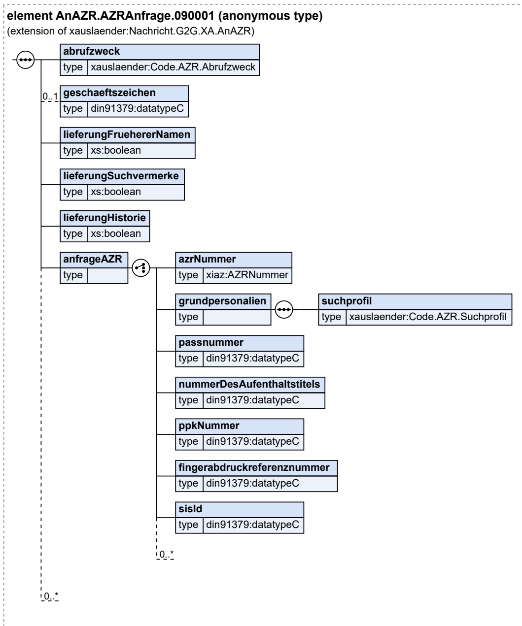
Abbildung 8.14. AnAZR.AZRAnfrage.090001
