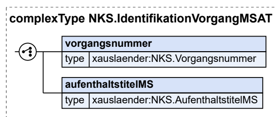
Abbildung 11.52. NKS.IndentifikationVorgangMSAT
